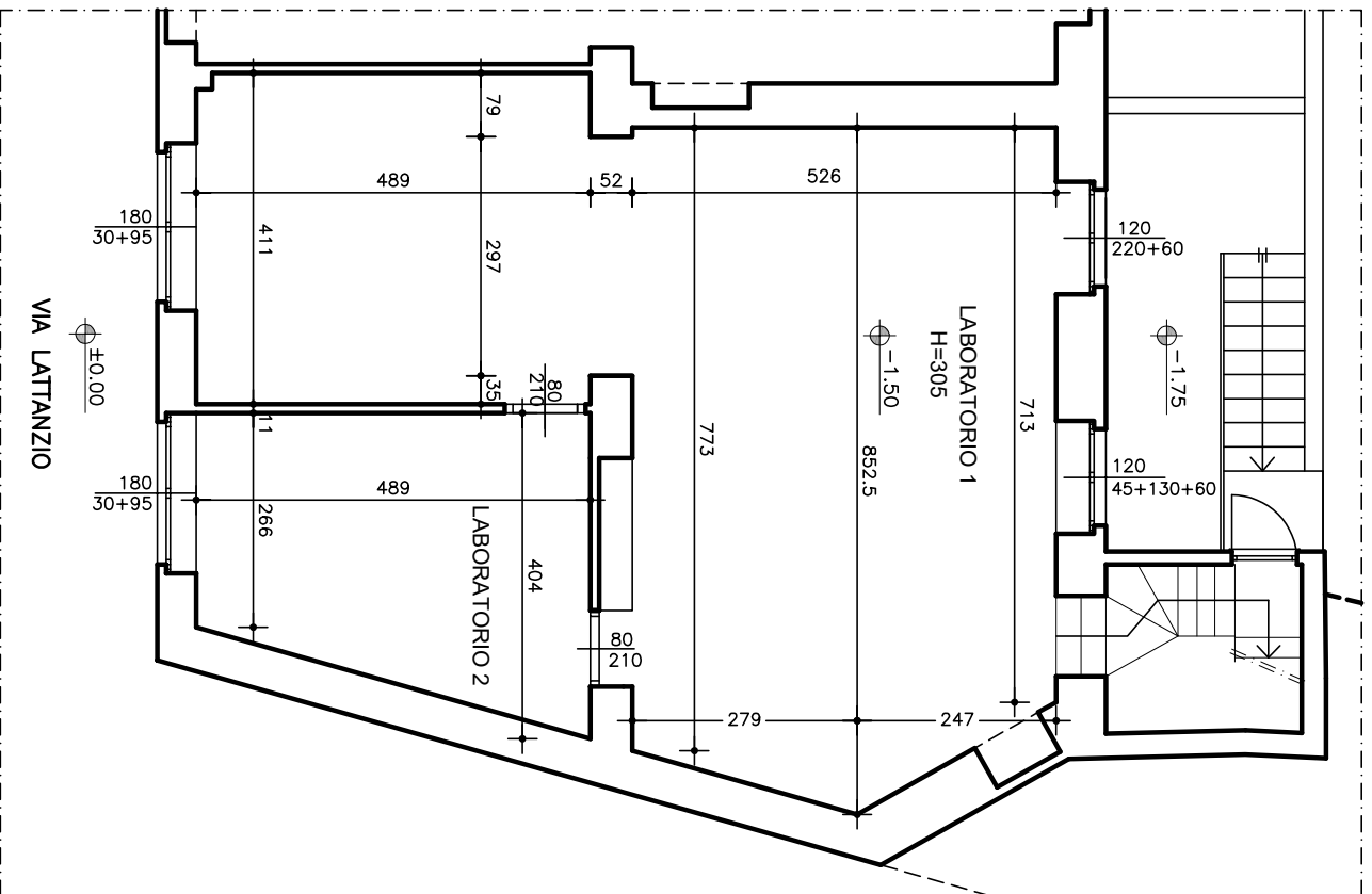
PIANTA PIANO RIALZATO
